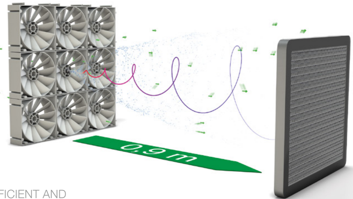
Vortex wall
